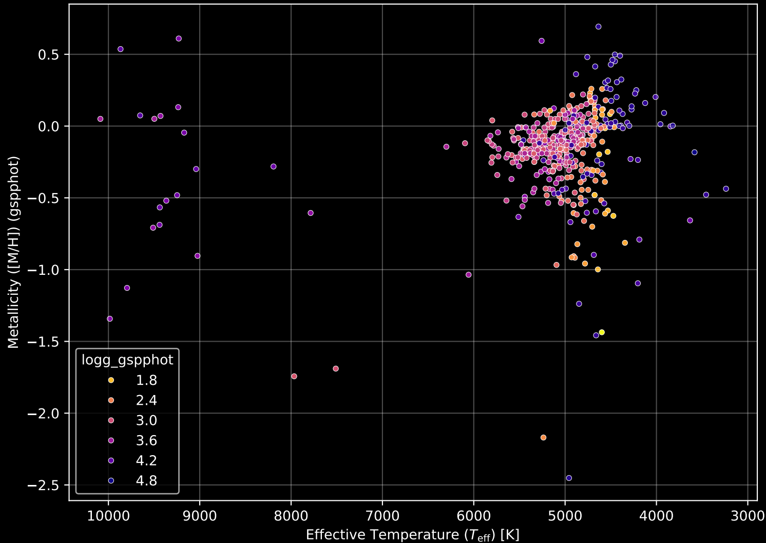
APOGEE DR17 Field: [180+08] Stellar Population Parameters (n= 494)
